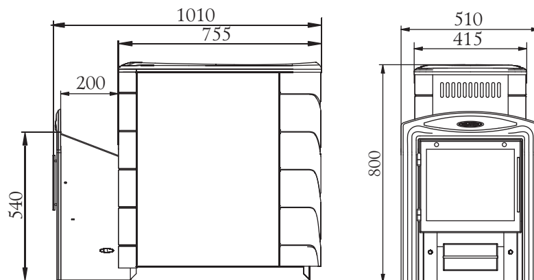
Bild 4. Ofenabmessungen «Tunguska XXL 2013 Vitra»
