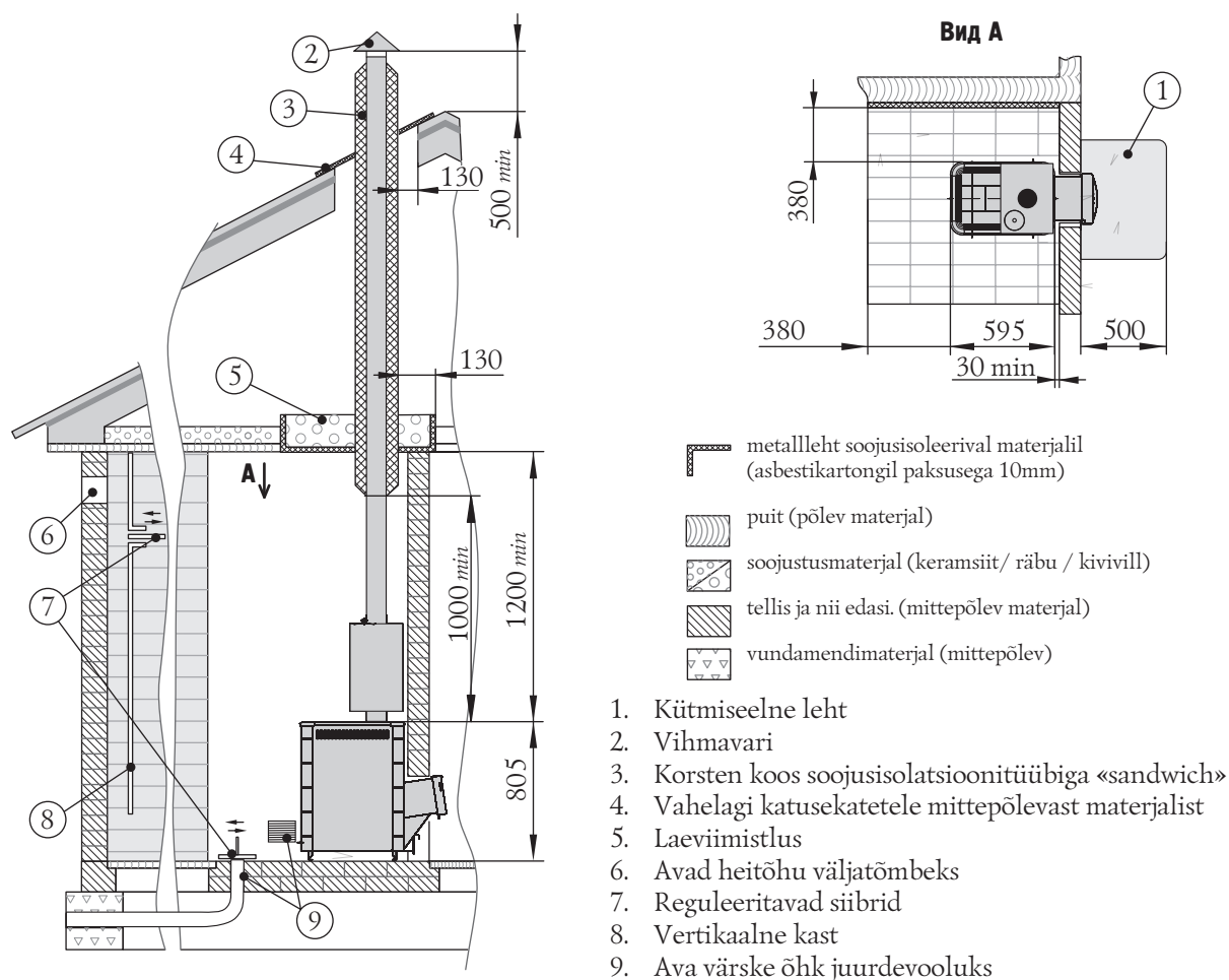
Joonis 7. Ahju paigaldamine ruumi mittepõlevast materjalist.
