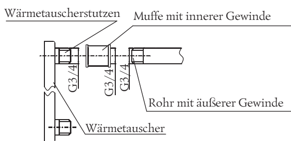
Bild 16. Muffenkupplung der Rohrleitung.
