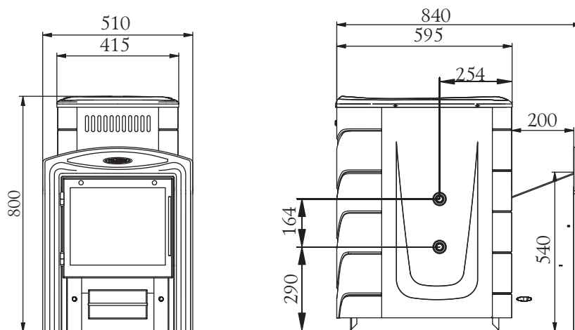
Bild 1. Ofenabmessungen «Tunguska 2011 Vitra»
