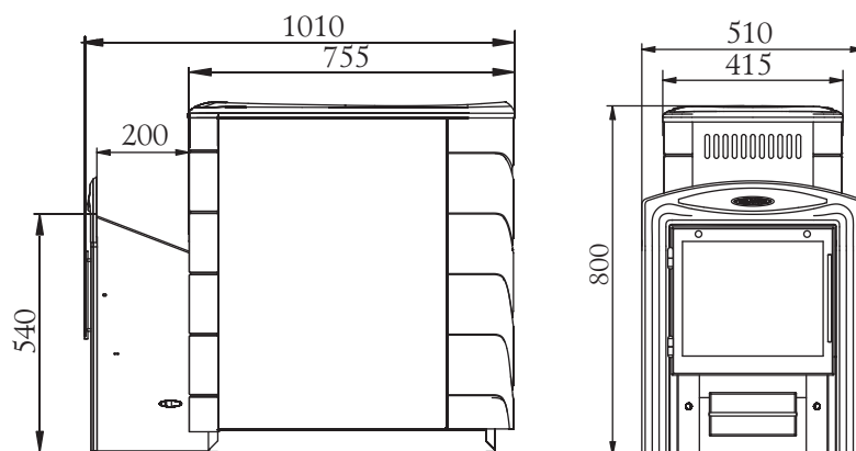
Рисунок 4. Габаритные размеры печи «Тунгуска XXL 2013 Витра».
