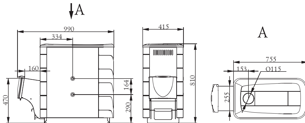
Bild 5. Ofenabmessungen «Tunguska XXL 2013».
