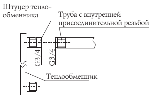
Рисунок 15. Присоединение трубопровода напрямую.
