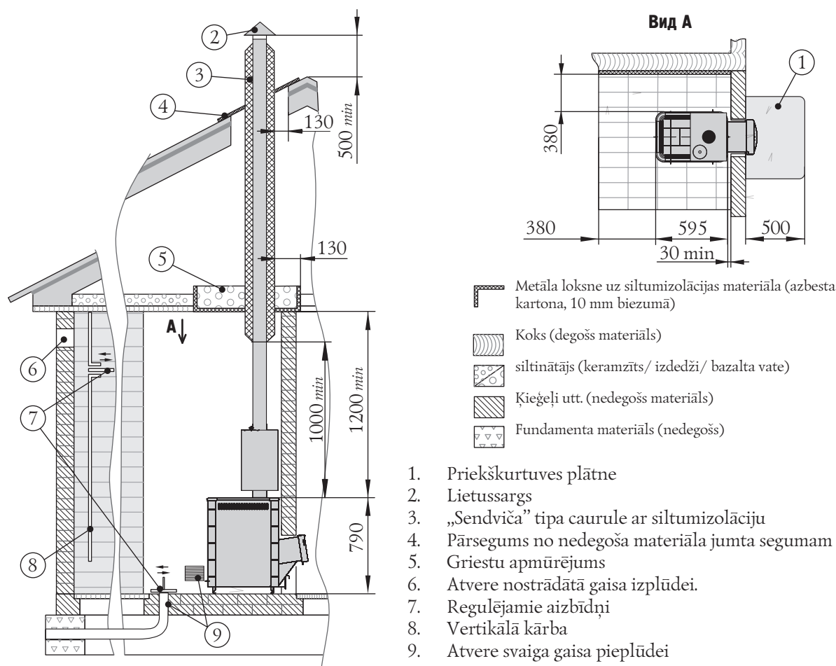
7. attēls. Krāsns montāža telpā no nedegoša materiāla
