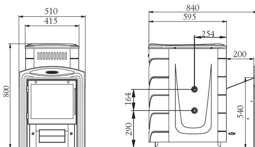
Paveikslėlis 1. Krosnies «Tunguska 2011 Vitra» gabaritiniai dydžiai
