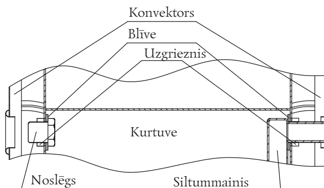
12. attēls. Krāsns „Tunguska” siltummaiņa un noslēgu demontāža
