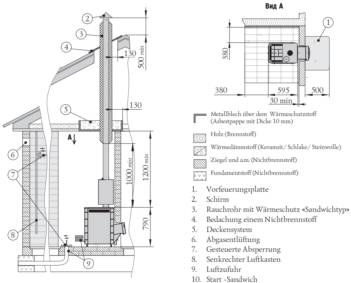
Bild 7. Ofenmontage im Raum aus einem Nichtbrennstoff
