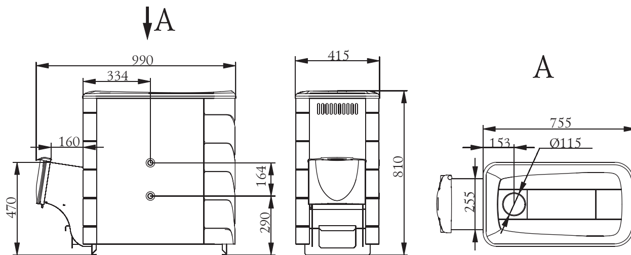
Joonis 5. Ahju «Tunguska XXL 2013» gabariitmõõtmed
