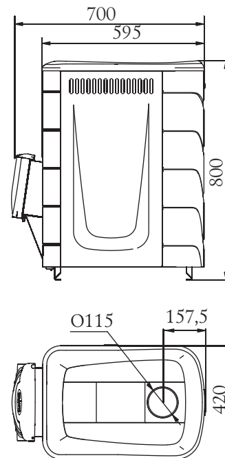
Bild 3. Ofenabmessungen «Tunguska 2011» mit dem kurzen Brennstoffkanal.
