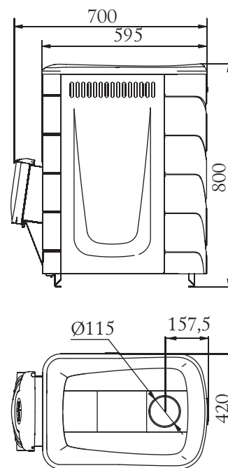
Рисунок 3. Габаритные размеры печи «Тунгуска 2011» с коротким топливным каналом.
