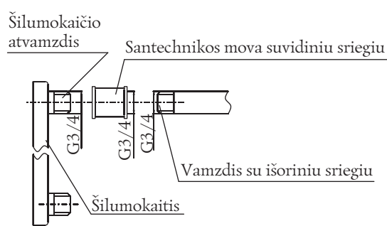
Paveikslėlis 16. Vamzdyno prijungimas per movą.
