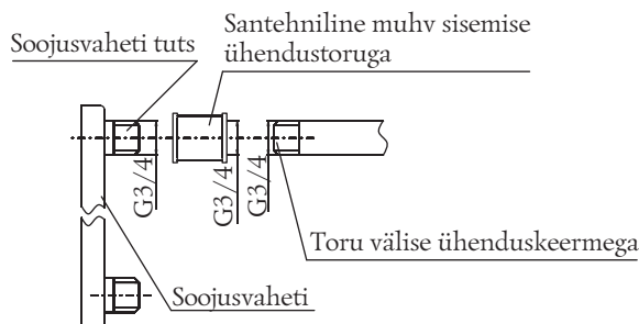
Joonis 16. Torustiku ühendamine muhvi kaudu.
