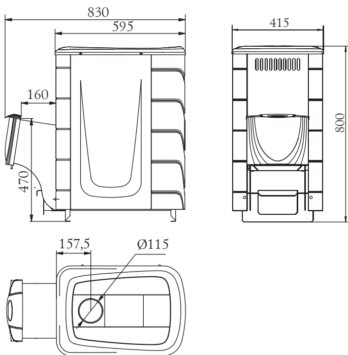
2. attēls. Krāsns «Tunguska 2011» gabarītu izmēri
