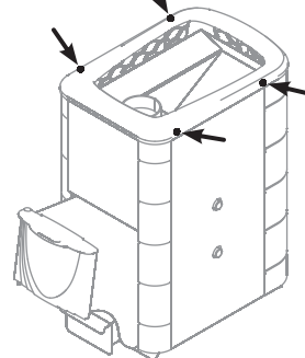
10. attēls. Krāsns „Tunguska” konvektora rāmja demontāža
