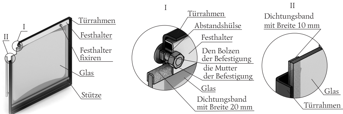
Bild 18. Befestigung des lichtdurchlässigen Schirms der Modelltür «Vitra»
