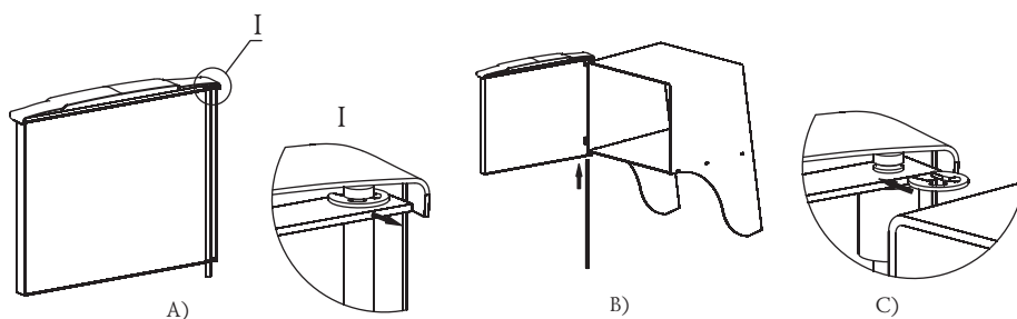
9. attēls. Durtiņu uzstādīšana krāsns «Tunguska» montāžas laikā
