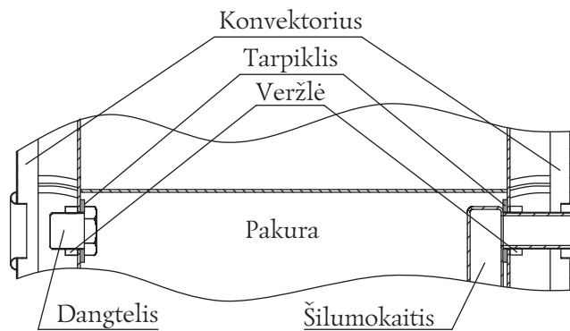
Paveikslėlis 12. Krosnies «Tunguska» šilumokaičio ir dangtelių demontavimas
