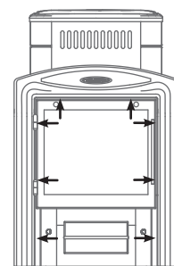
8. attēls. Durtiņu ar rāmi demontāža, «Vitra» krāsns modeļa montāžas laikā
