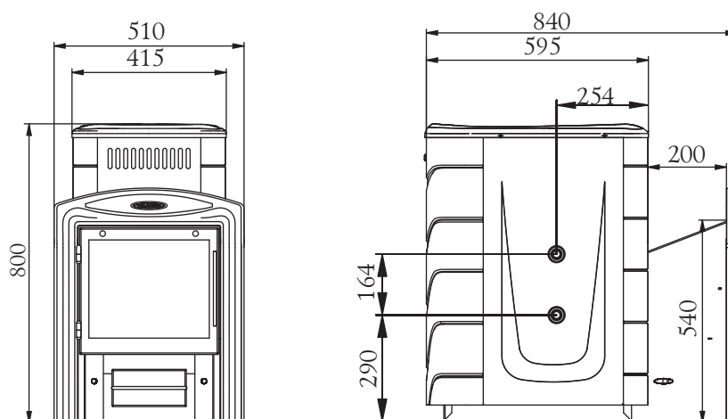
1. attēls. Krāsns «Tunguska 2011 Vitra» gabarītu izmēri
