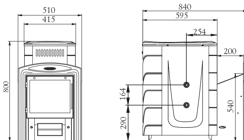
Joonis 1. Ahju «Tunguska 2011 Vitra» gabariitmõõtmed
