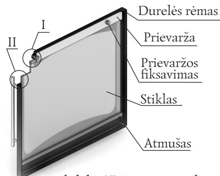
Paveikslėlis 17. Permatomo ekrano durelyje taisymas modelyje «Vitra»
