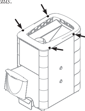
Paveikslėlis 10. Krosnies «Tunguska» konvektoriaus rėmelio demontavimas
