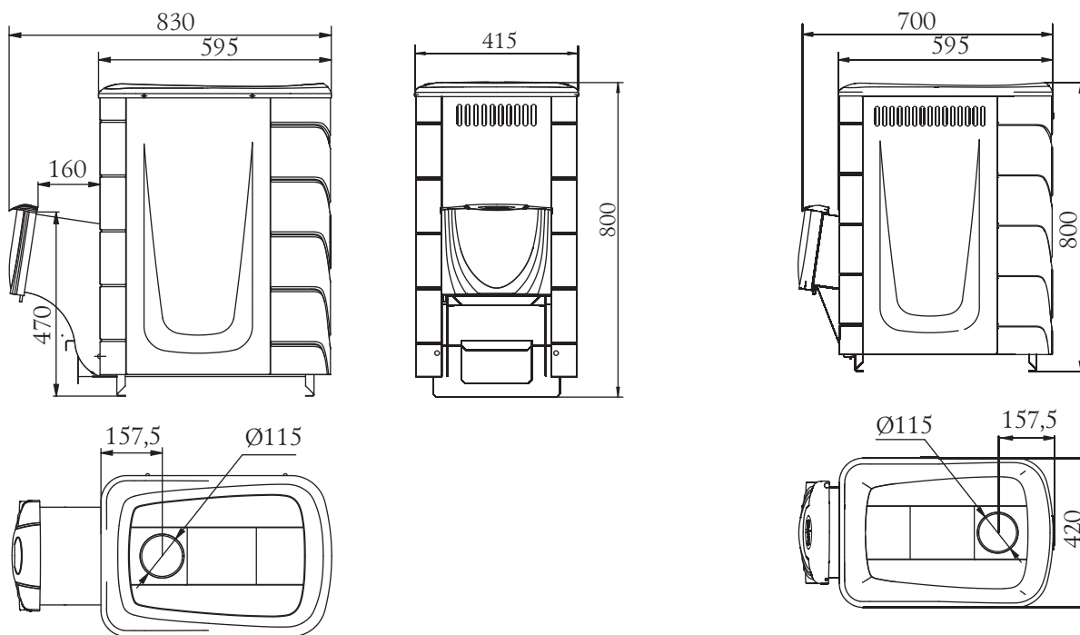
Paveikslėlis 3. Krosnies «Tunguskos 2011» trumpas kuro kanalo.
