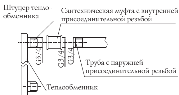
Рисунок 16. Присоединение трубопровода через муфту.
