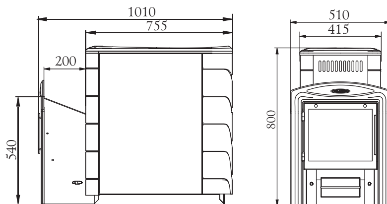
Joonis 4. Ahju «Tunguska XXL 2013 Vitra» gabariitmõõtmed
