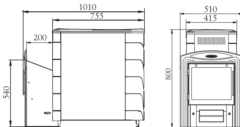
Paveikslėlis 4. Krosnies «Tunguska XXL 2013 Vitra» gabaritiniai
