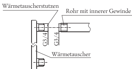
Bild 15. Direkte Verbindung der Rohrleitung.
