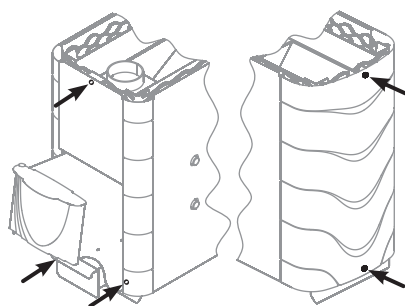
11. attēls. Krāsns „Tunguska” konvektora demontāža
