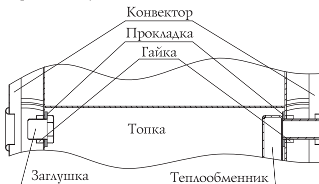
Рисунок 12. Демонтаж теплообменника и заглушек печи.
