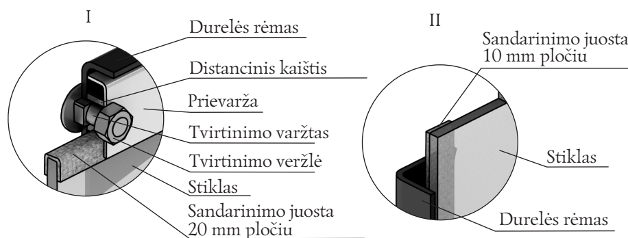
Paveikslėlis 18. Permatomo ekrano durelyje taisymas modelyje «Vitra»
