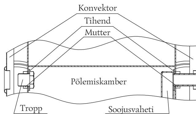
Joonis 12. Ahju «Tunguska» soojusvaheti ja demonteerimine
