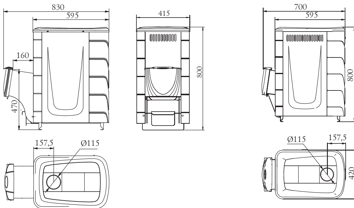
Joonis 3. Ahju «Tunguska 2011» lühike kutuse kanal.
