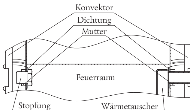
Bild 12. Demontage des Wärmetauschers und der Ofenklappen «Tunguska»
