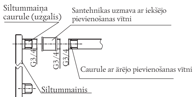
16. attēls. Cauruļvada pievienošana caur uznavu
