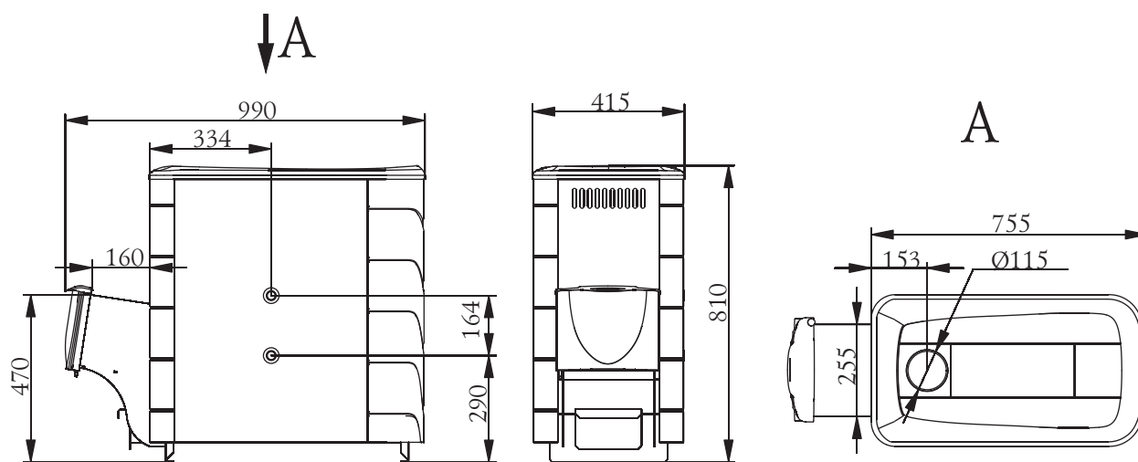
Рисунок 5. Габаритные размеры печи «Тунгуска XXL 2013».
