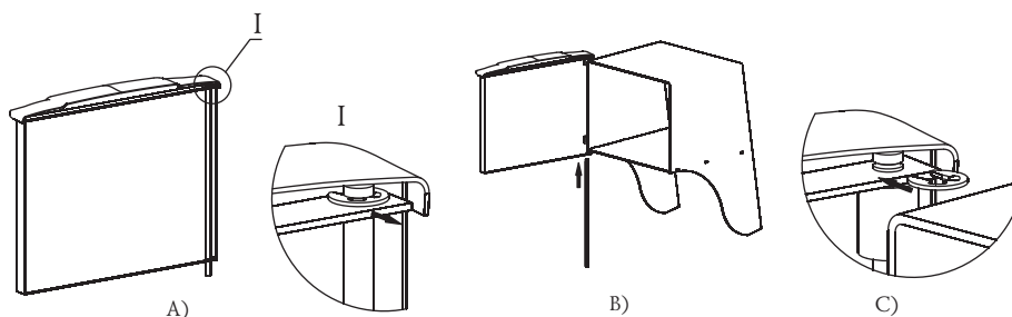
Joonis 9. Ukse paigaldamine ahju «Tunguska» monteerimise korral
