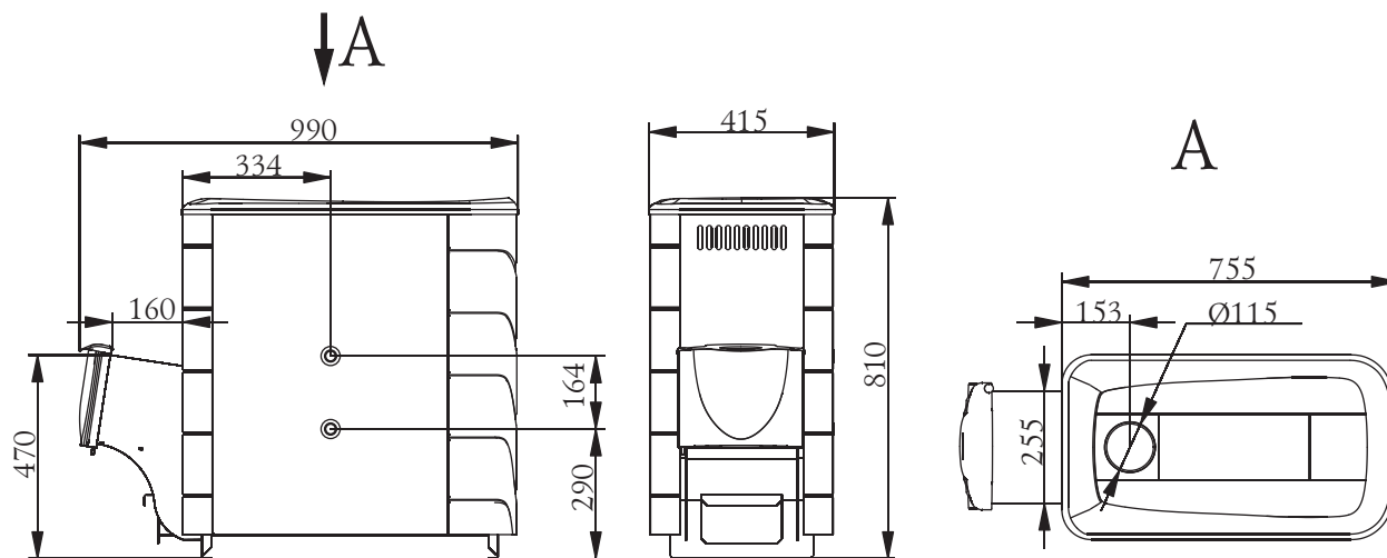
Paveikslėlis 4. Krosnies «Tunguska XXL 2013 Vitra» gabaritiniai
