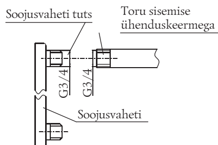
Joonis 15. Torustiku ühendamine otse
