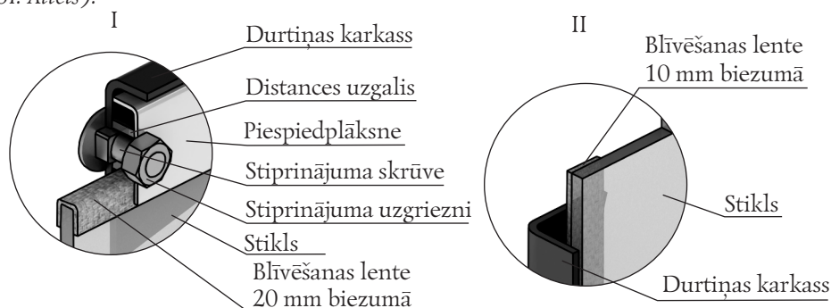
18. attēls. Gaismaurlaidīgā ekrāna stiprināšana «Vitra» modeļa durtiņās
