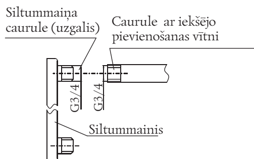
15. attēls. Cauruļvada tiešā pievienošana
