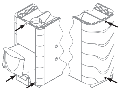
Paveikslėlis 11. Krosnies «Tunguska» konvektoriaus demontavimas
