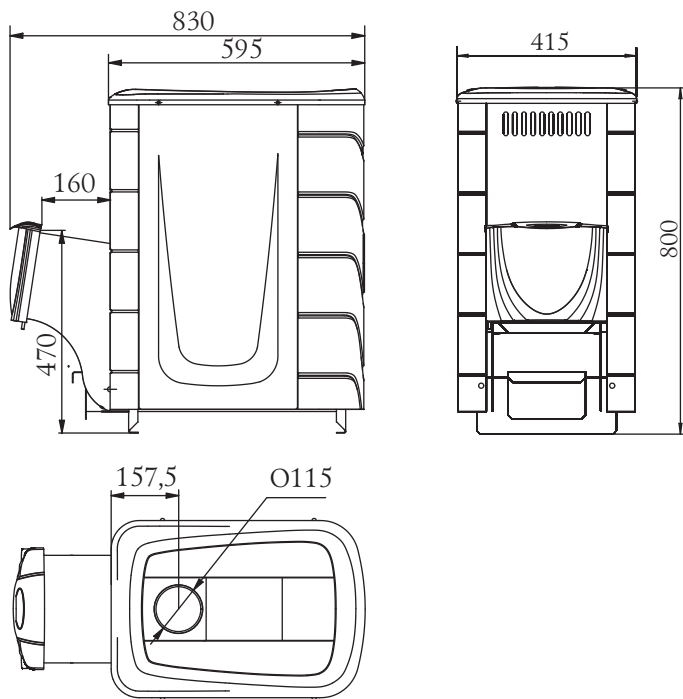
Bild 2. Ofenabmessungen «Tunguska 2011»
